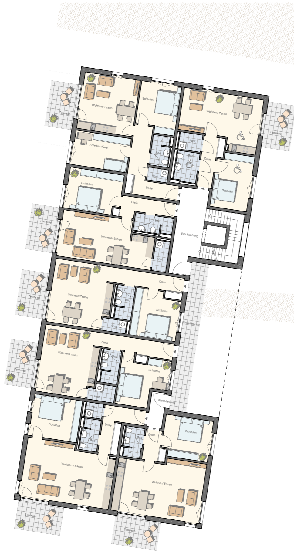
EG - Gebäude D 1:200
